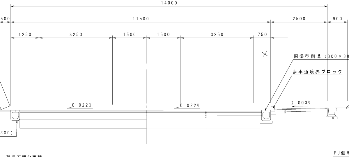
標準断面図 S=1:100
