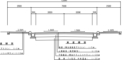
標準断面図 S=1:100
