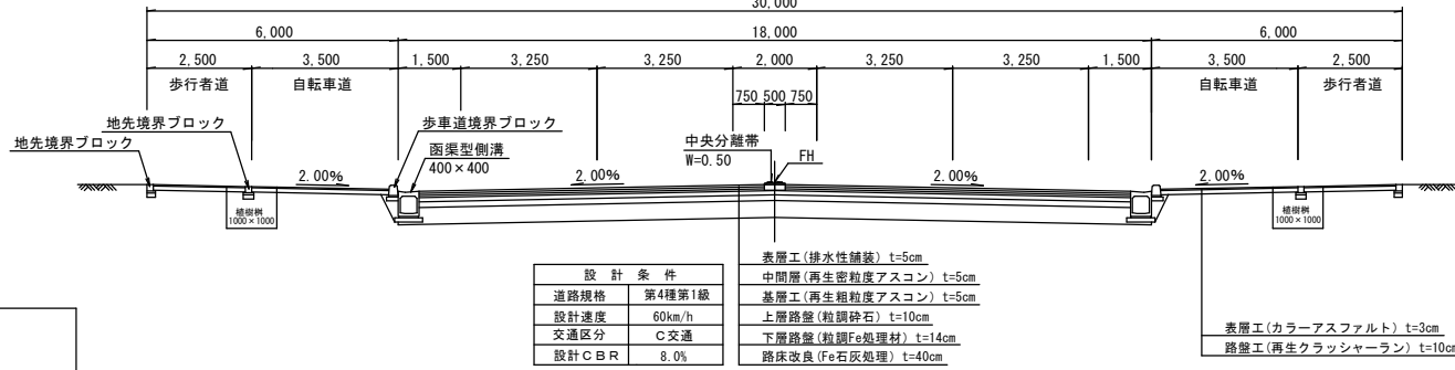
標準断面図 S=1:200
