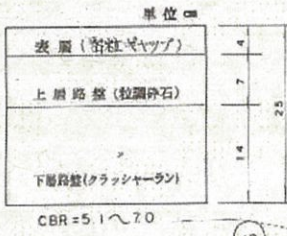
舗装構造図
