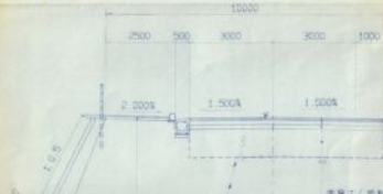
標準断面図 S=1:100
