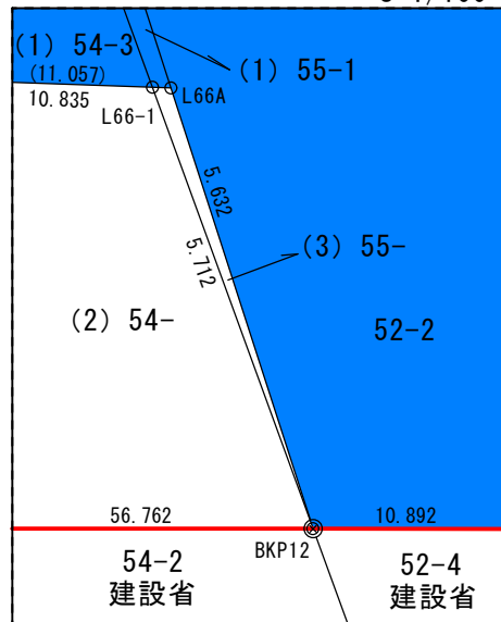
拡大図 A S=1/100
