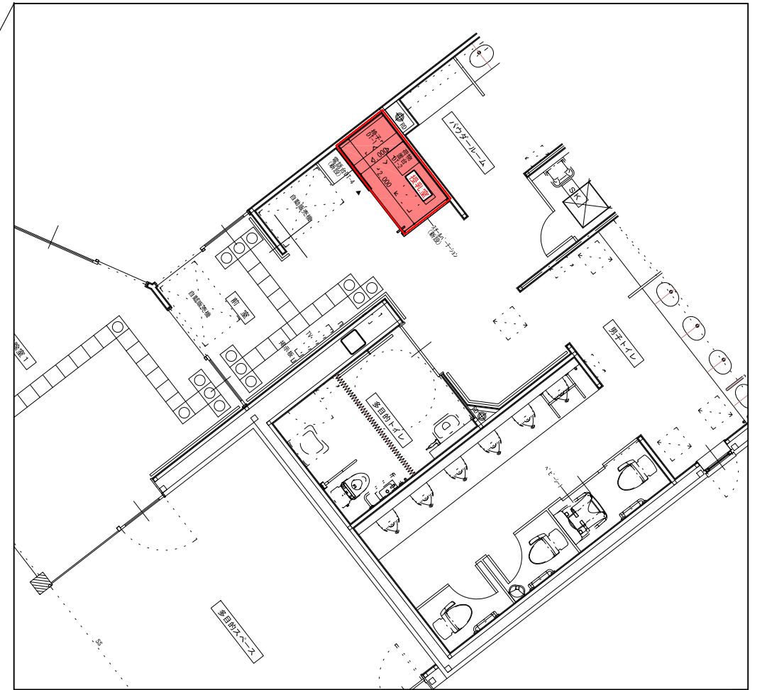
拡大図 S=1:100
